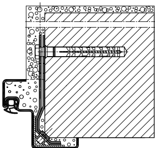
Mit Schraubanker in Laibung
