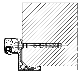
Verdeckte Schraubmontage
