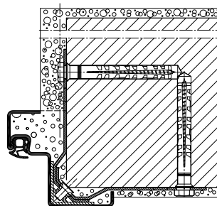
Schraubanker beidseitig
